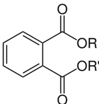
Figur 1. Generell struktur av ftalater. R och R' är allmänna platsbyllare.
