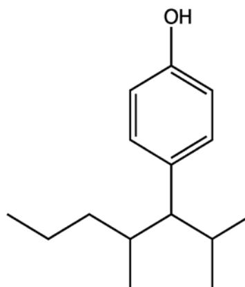
Figur 2. Generell struktur av nonylfenol.
